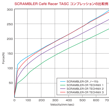
ダイノテストと実走行テストで、様々なライディングフィールドのセッティングデータをチャート化し仕様を決定しています。
