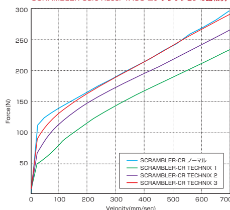
SCRAMBLER Café Racer TASC コンプレッションの比較例
