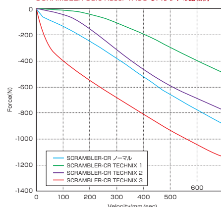
SCRAMBLER Café Racer TASC リバウンドの比較例
